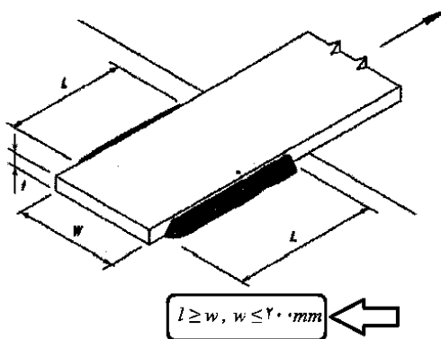
شکل ۴-۹-۲-۱۰ جوش گوشه در انتهای تسمه‌های کششی
